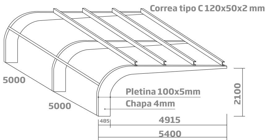
🔍 DETALLE BRAZO APARCAMIENTO (mm)
